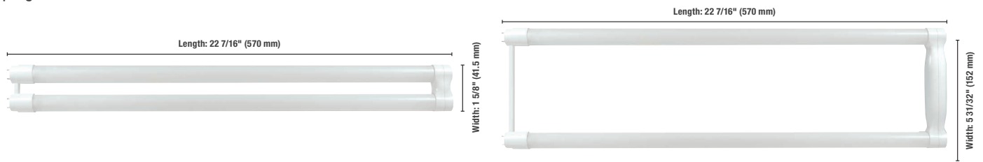
U-Bent U1
